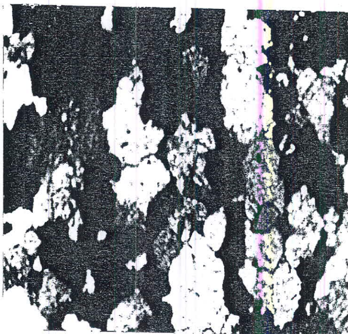
عکس شماره (۸-۴) نشانگر بافت موزائیکی تا بعضا برشی را همراه با بلورهای کلسیتی و دولومیتی می باشد. بزرگنمایی 10 \times 7/3
